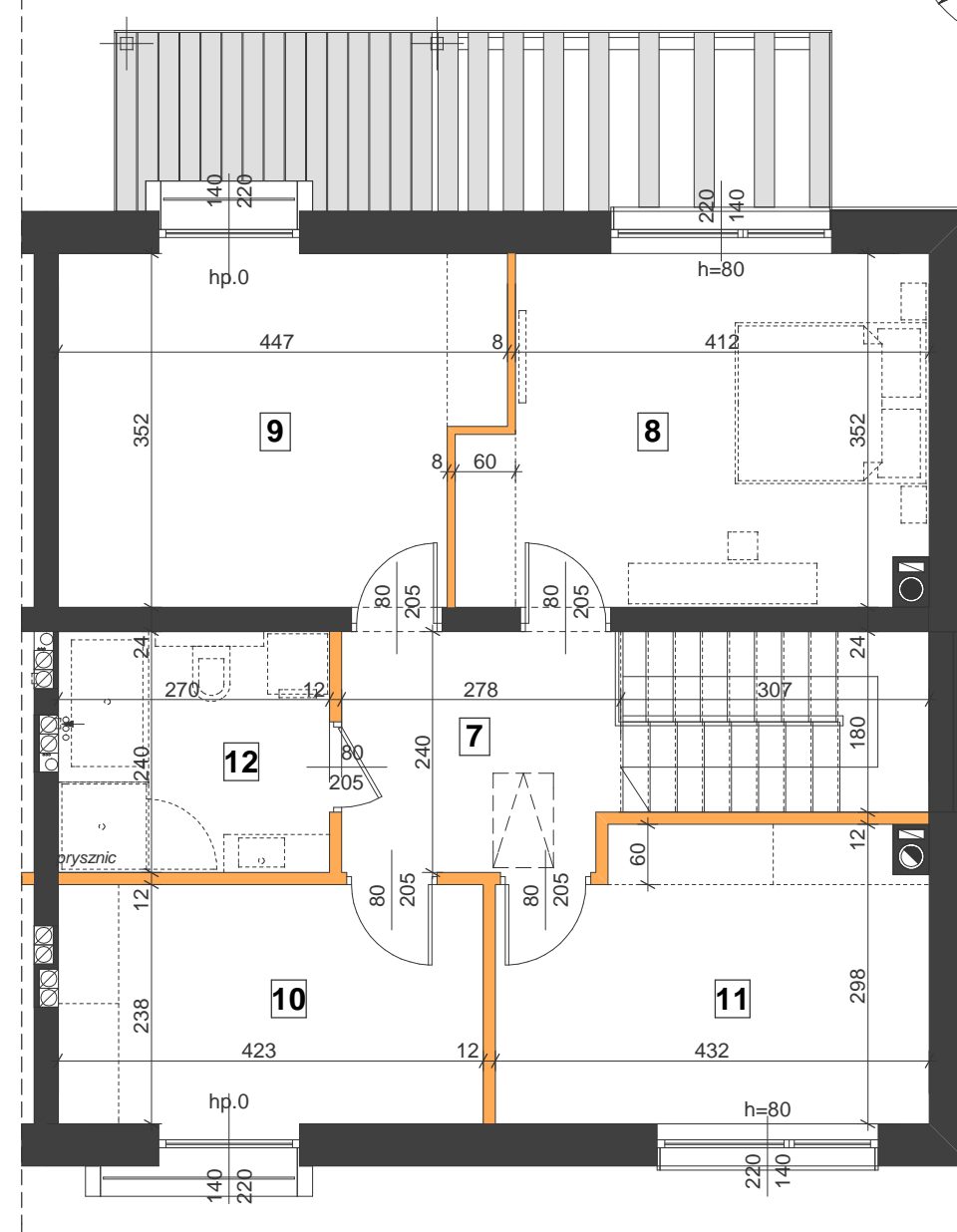
plan piętra
