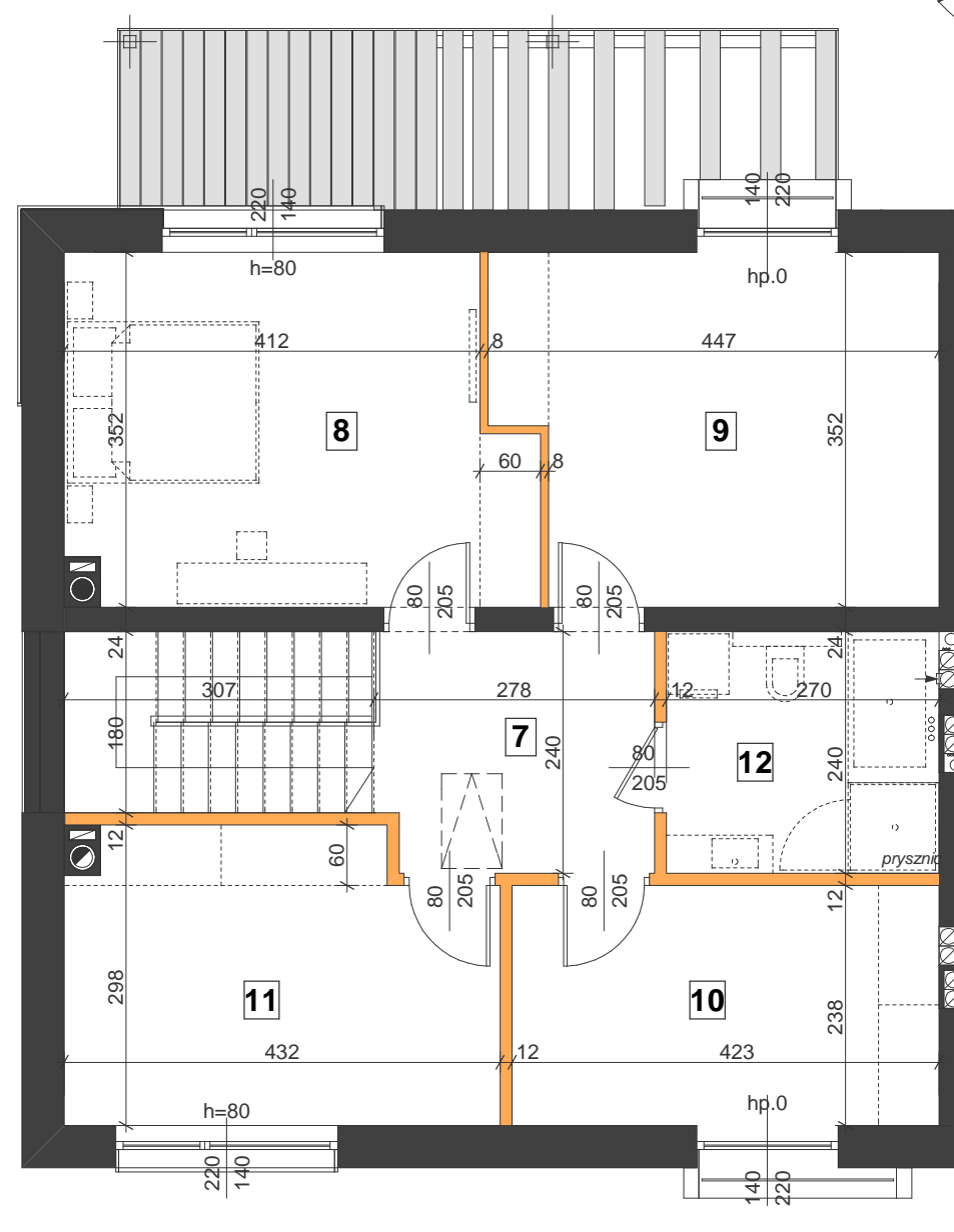
plan piętra
