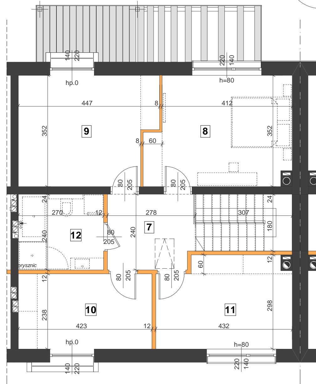
plan piętra
